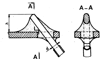
Obr. 7. Pájení — příklad normálního provedení
